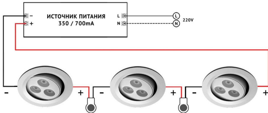
Схема последовательного подключения нескольких светильников к источнику питания с выходным током 350 / 700mA
